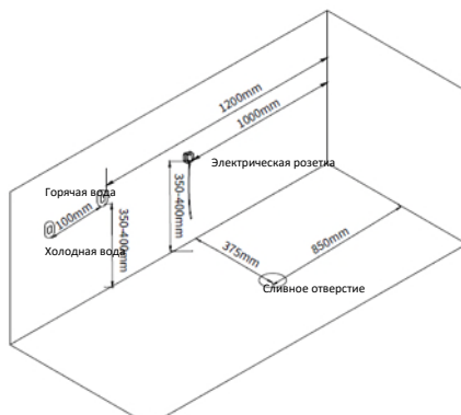
Схема расположения точек подключения
